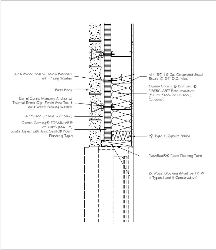
21 FOAMULAR® XPS, Steel Stud Jamb
