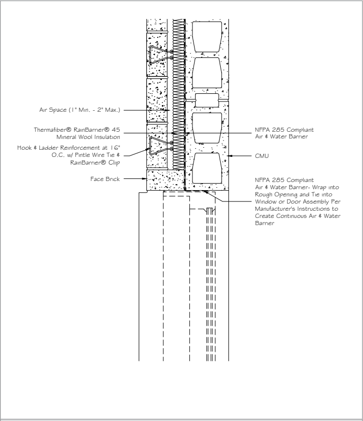
48 Thermafiber® MW, CMU Jamb
