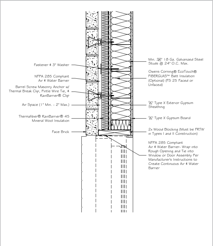
40 Thermafiber® MW, Steel Stud Jamb
