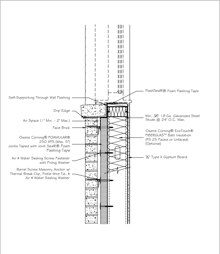
24 FOAMULAR® XPS, Steel Stud Sill
