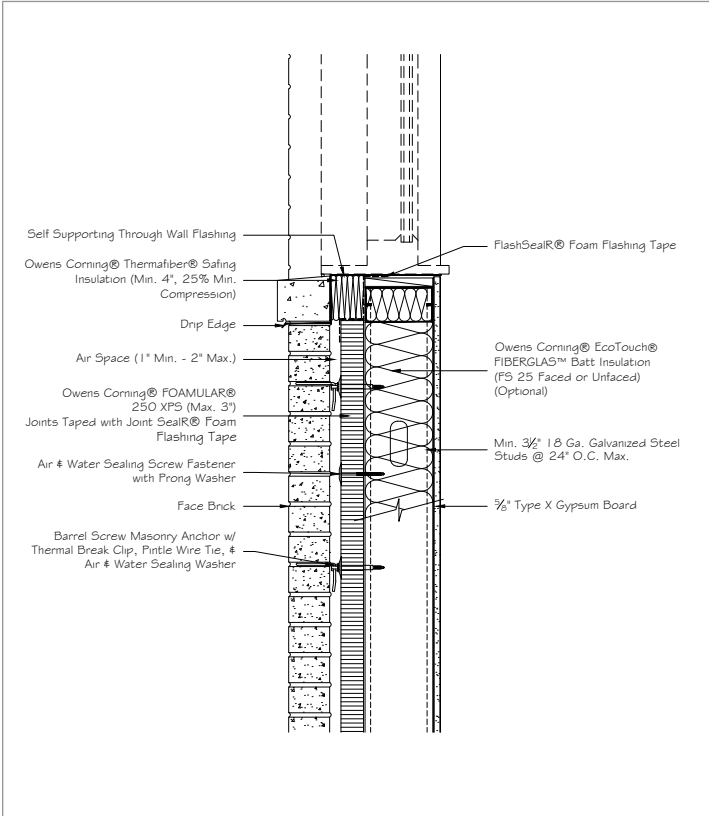
23 FOAMULAR® XPS, Steel Stud Sill
