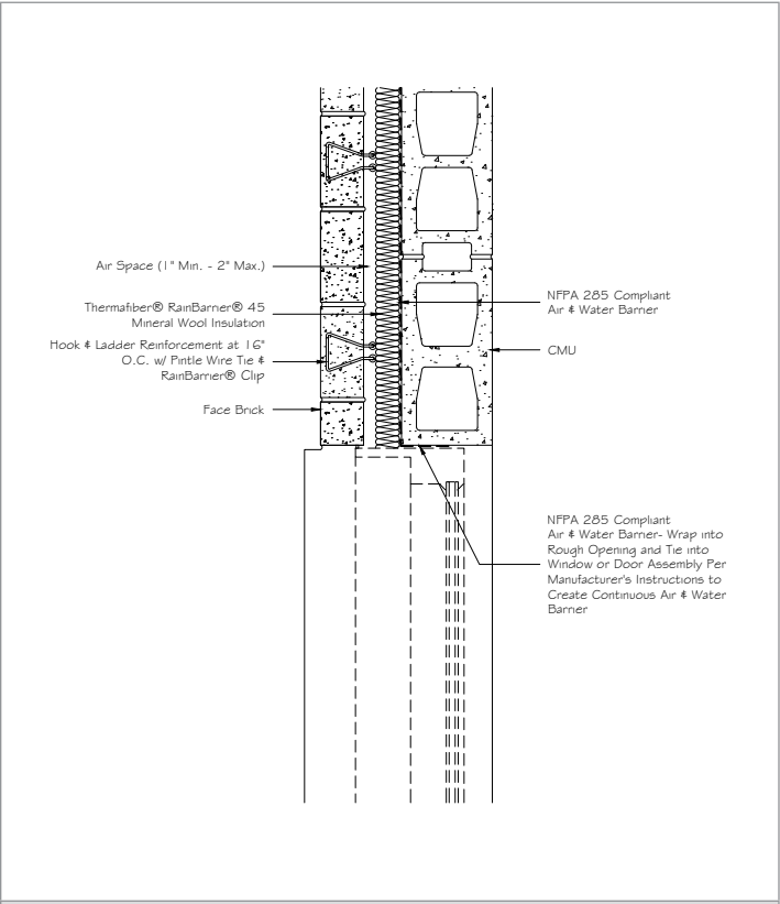
46 Thermafiber® MW, CMU Jamb
