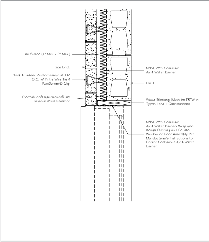
47 Thermafiber® MW, CMU Jamb
