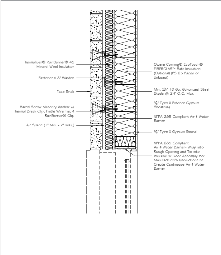
39 Thermafiber® MW, Steel Stud Jamb
