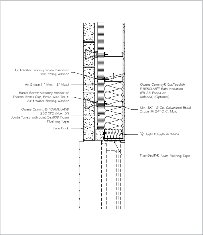
22 FOAMULAR® XPS, Steel Stud Jamb
